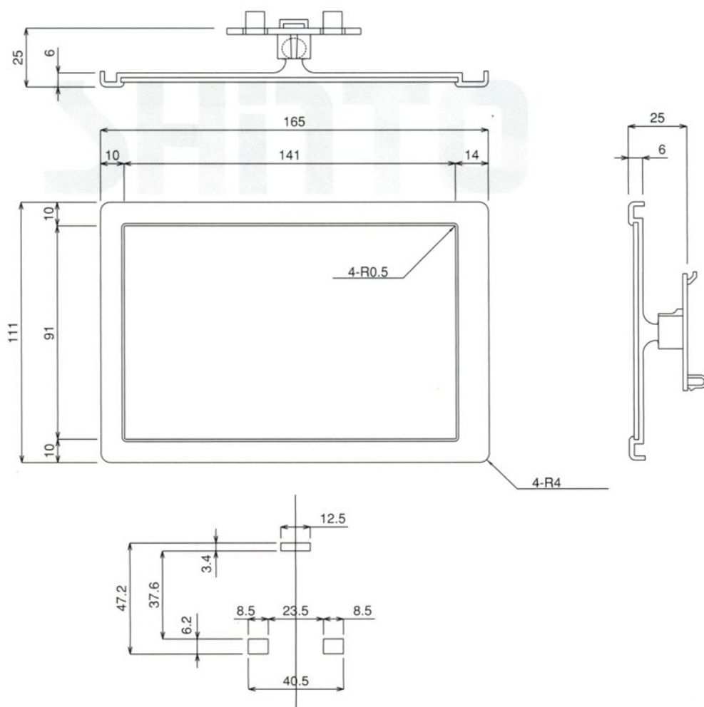
パネル切欠き寸法
