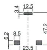
パネル穴明寸法
