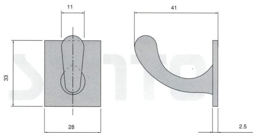
SDフック本体
