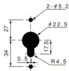
パネル穴明け寸法
