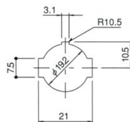
パネル穴明け寸法・位置 (CL-01,03,04,05)
