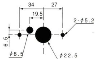
パネル穴明け寸法
