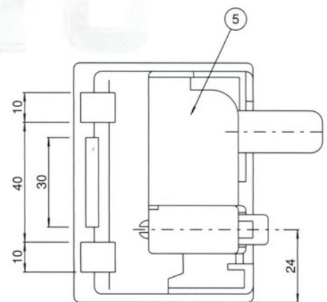
背面図
