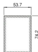
パネル穴寸法 S=1/2
